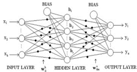
Gambar 2 : Jaringan Syaraf Tiruan Feed-Forward
